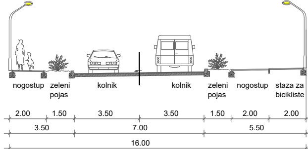
POPREČNI PRESJEK B-B ZA SABIRNU ULICU SU
