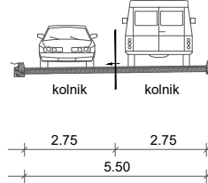
POPREČNI PRESJEK C-C ZA INTERNU ULICU IU3
