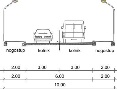
POPREČNI PRESJEK C-C ZA INTERNU ULICU IU3
