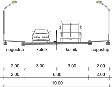
POPREČNI PRESJEK B-B ZA SABIRNU ULICU SU
